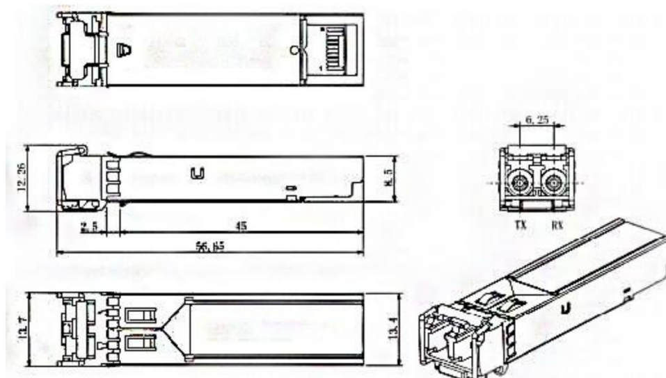
Figura 6. Desenho Mecânico
