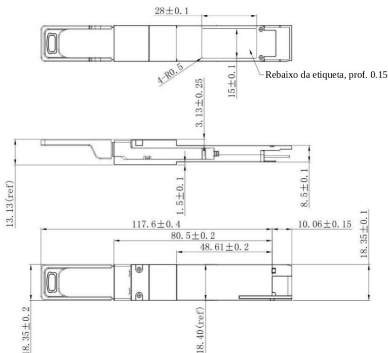
Figura 2. Dimensões do módulo. Cotas em mm, tolerância de \pm 0,2 mm salvo indicação em contrário
