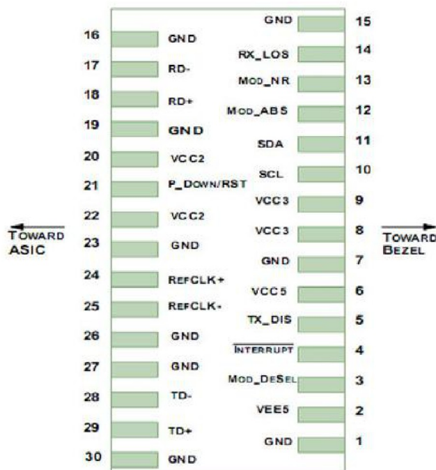
Figura 1. Atribuição dos pads do conector XFP (Toward ASIC: lado do host; Toward Bezel: lado do painel frontal)
