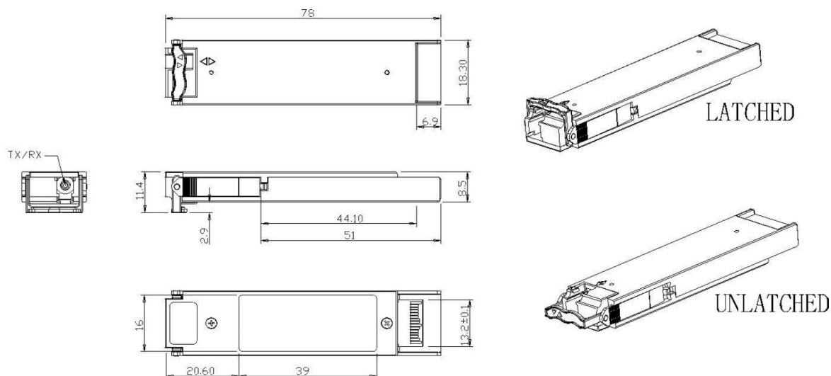
Figura 2. Dimensões do módulo (à direita, trava fechada/LATCHED e aberta/UNLATCHED). Cotas em mm, tolerância de \pm 0,2 mm salvo indicação em contrário
