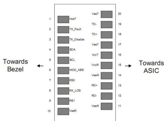
Figura 1. Atribuição dos pinos do SFP+ (Towards Bezel: lado do painel; Towards ASIC: lado do host)
