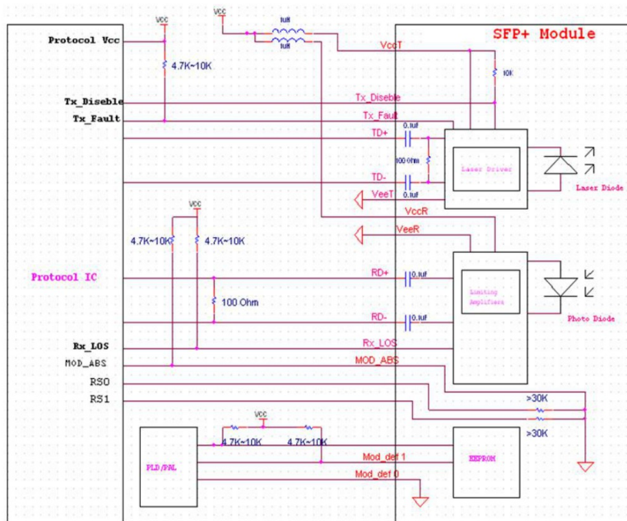
Figura 2. Circuito de interface recomendado (host e módulo SFP+)
