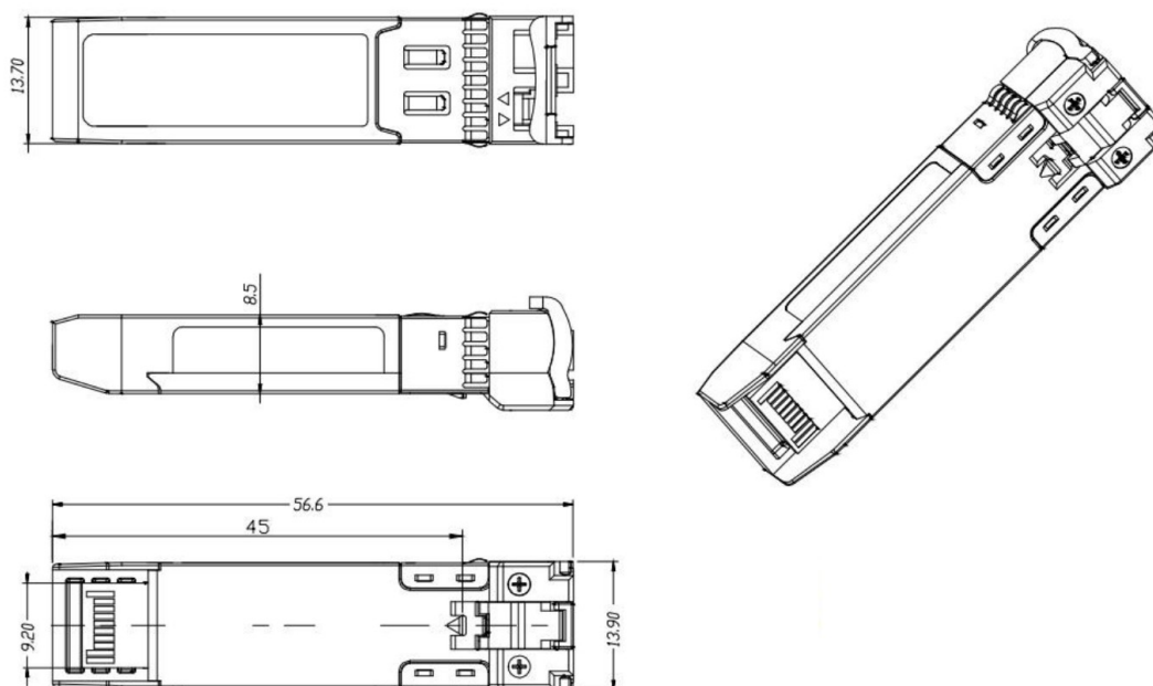
Figura 3. Dimensões do módulo. Cotas em mm, tolerância de \pm 0,2 mm salvo indicação em contrário
