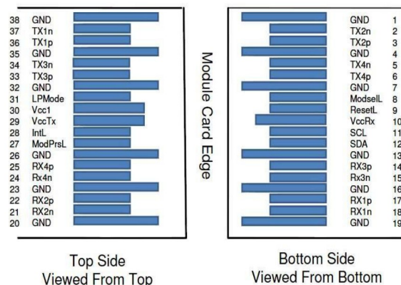
Figura 1. Conector de 38 pinos compatível com QSFP MSA
