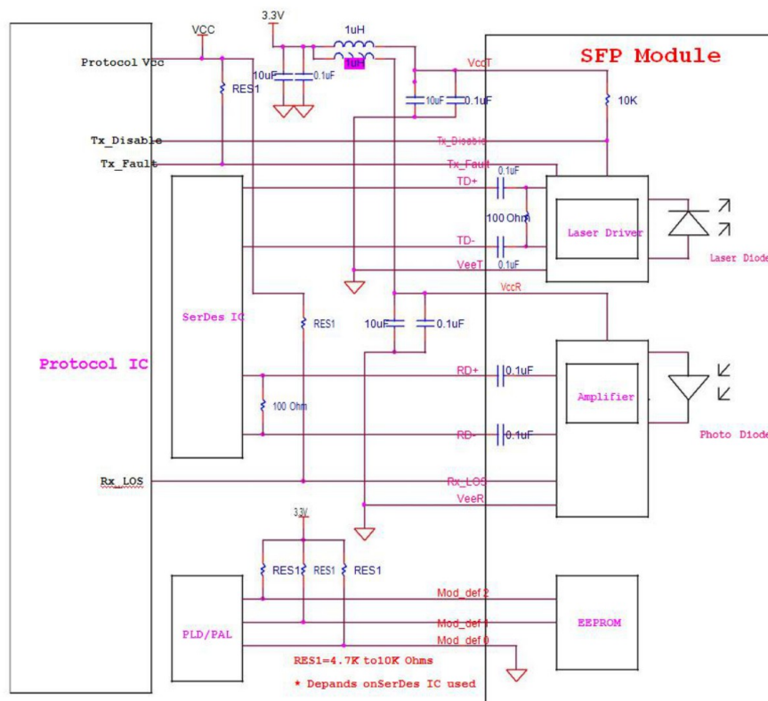
Figura 3. Circuito esquemático recomendado
