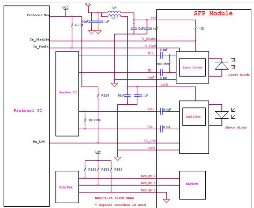
Figura 1. Circuito esquemático de interface com o host
