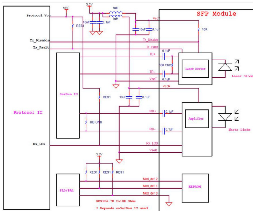
Figura 1. Circuito esquemático de interface com o host
