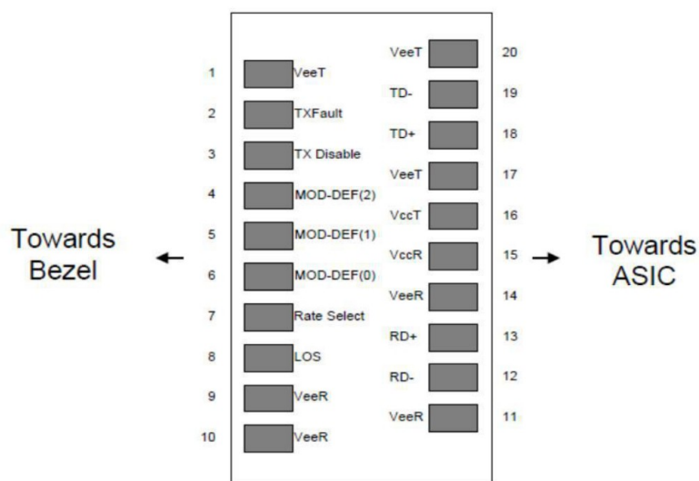
Figura 2. Pinagem do conector SFP (vista pelo topo da placa)
