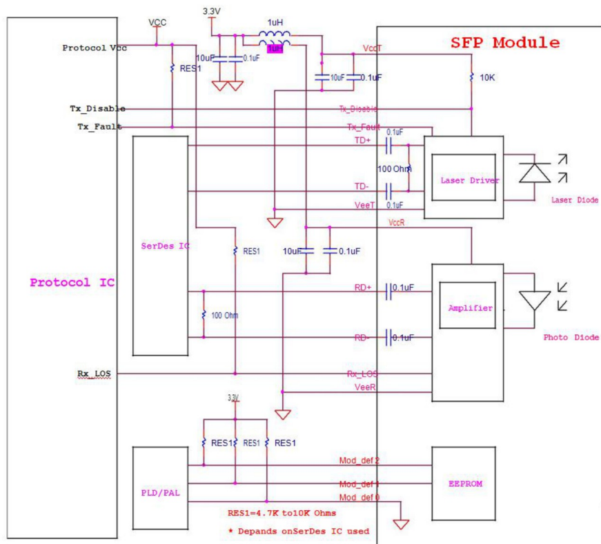
Figura 3. Circuito esquemático recomendado
