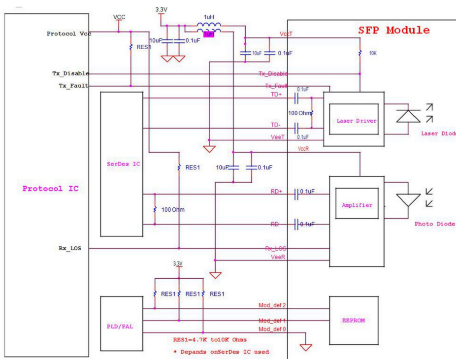
Figura 2. Circuito de aplicação típico
