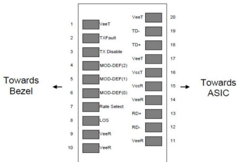
Figura 1. Pinagem do conector SFP (vista pelo topo da placa)
